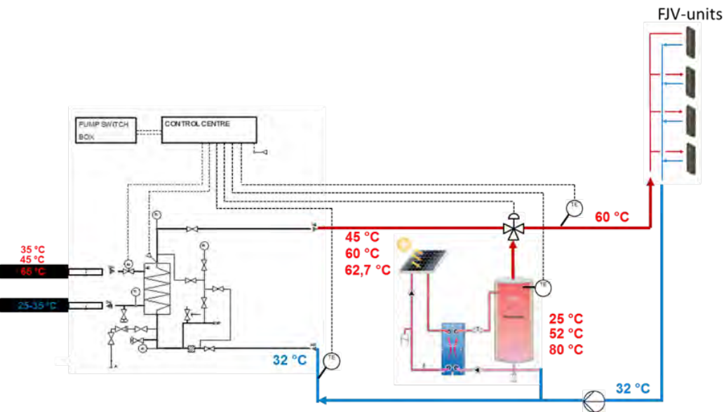
Figur 57 - Principskitse af et solvarmeanlæg i samspil med fjernvarme og installation af FJV-units (Kilde: Alfa Laval)
