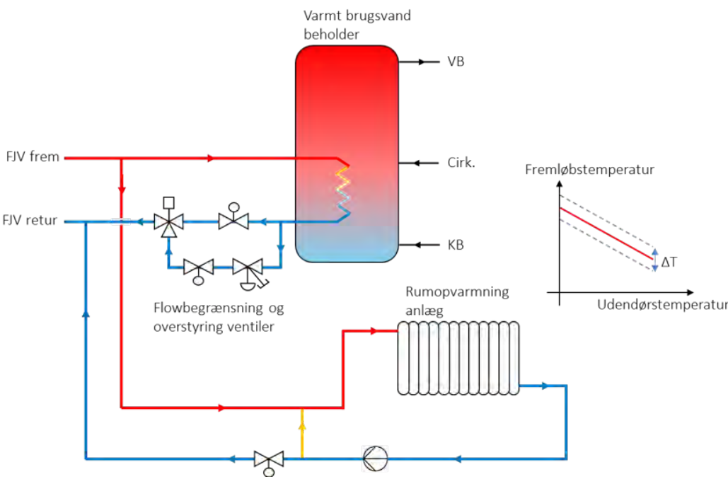
Figur 36 - Principskitse af rumopvarmning og varmt brugsvand system med lagring muligheder
