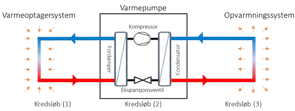
Figur 18 - Principskitse af et varmepumpeanlæg
