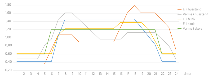
Figur 4: Døgnbaserede kurver (normaliseret) for typisk husstandsforbrug af el og varme, samt offentlige institutioners og butikkers forbrug af el og varme, der bl.a. viser spidslasterperioder.
